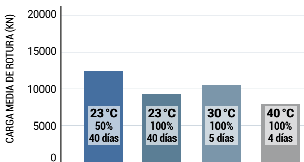
RESISTENCIA A LA FLEXIÓN DEL REFUERZO FRP EN FUNCIÓN DE LA TEMPERATURA, LA HR Y LOS DÍAS DE EXPOSICIÓN
