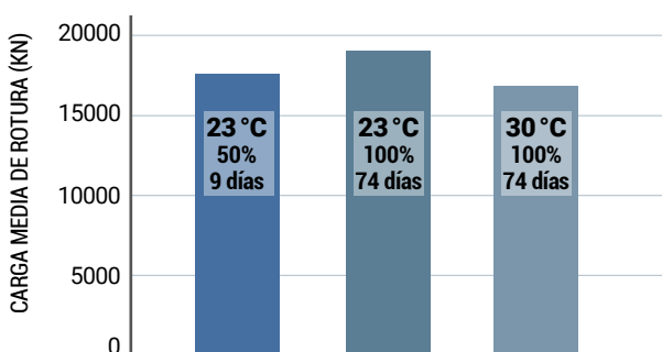
RESISTENCIA A LA FLEXIÓN DEL REFUERZO FRCM EN FUNCIÓN DE LA TEMPERATURA, LA HR Y LOS DÍAS DE EXPOSICIÓN
