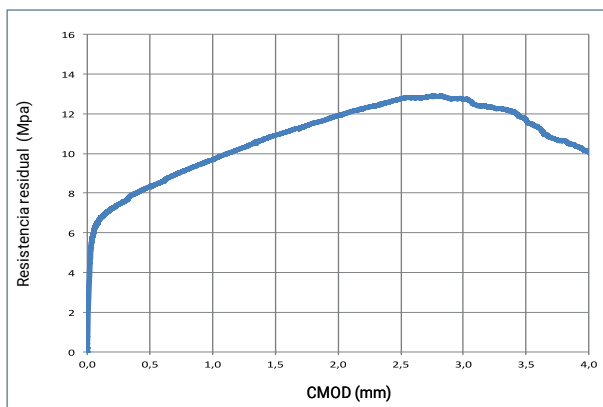
Micro Gold FCC: resistencia a la flexión residual EN 14651
