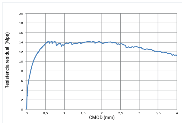
Micro Gold Steel: resistencia a la flexión residual EN 14651
